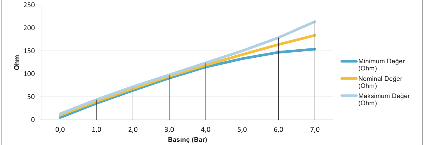
7 Bar Basınca Göre Karakteristik Eğriler (Devam)
